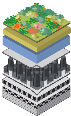
Opbouw Nophadrain Lichtgewicht Waterbufferingsdaksysteem met ND 6+1v
