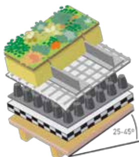
Compositie Nophadrain Extensief Groendaksysteem - steil dak
