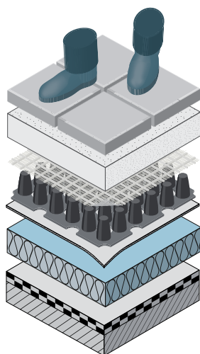
Opbouw met ND TRASDRAIN® 200sv Drainagesysteem
