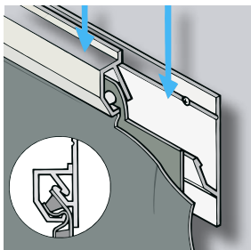
ND „Clic“ Systeem-Profiel
